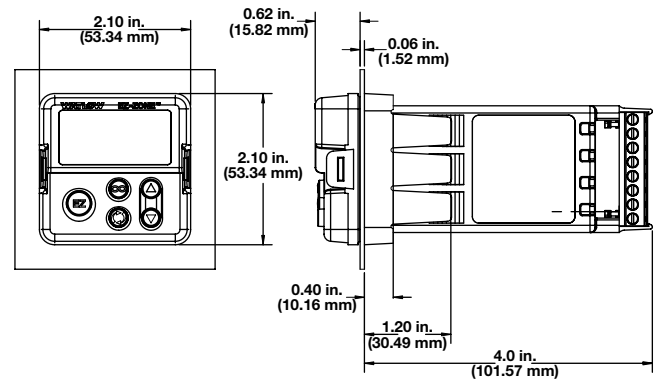
EZ-ZONE PM \frac{1}{16} DIN
