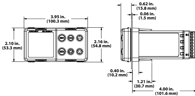
EZ-ZONE PM 1/8 DIN Horizontal
