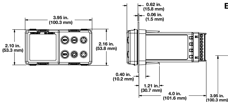
EZ-ZONE PM \frac{1}{8} DIN - Horizontal
