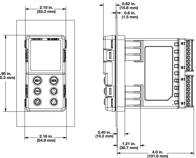
EZ-ZONE PM \frac{1}{8} DIN - Vertical
